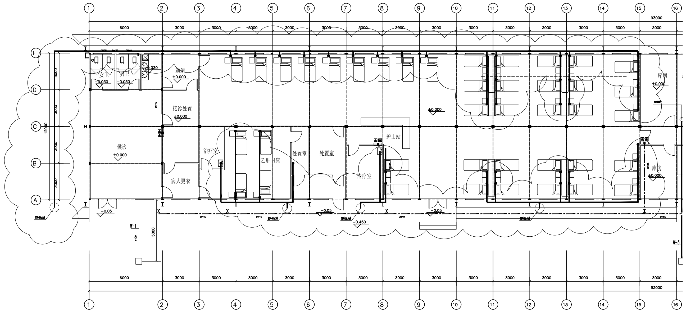
一层给排水平面图 1:100
